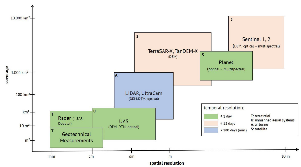
Abb. 3: Monitoring Methoden unter Berücksichtigung der räumlichen und zeitlichen Auflösung sowie Abdeckung.
