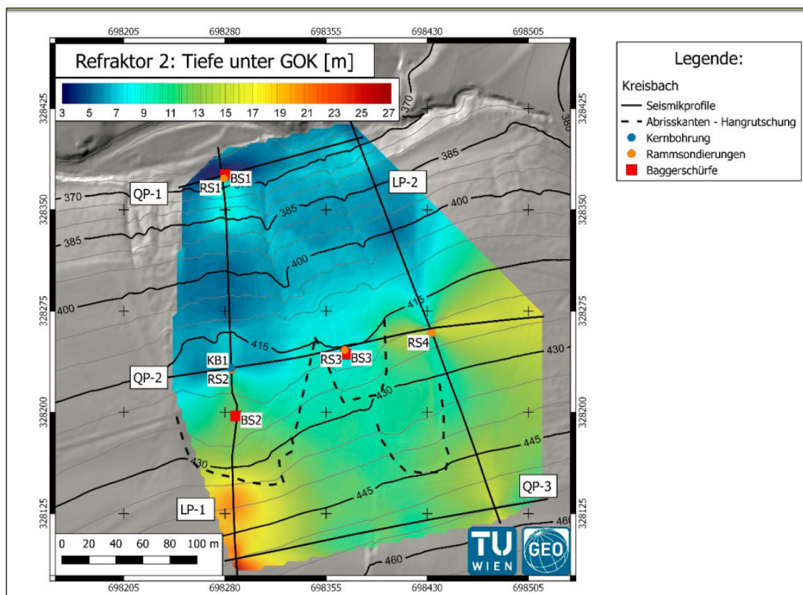
Abb. 8: Karte der interpolierten Tiefe unter GOK des zweiten Refraktors auf Basis der einzelnen Messprofile.
