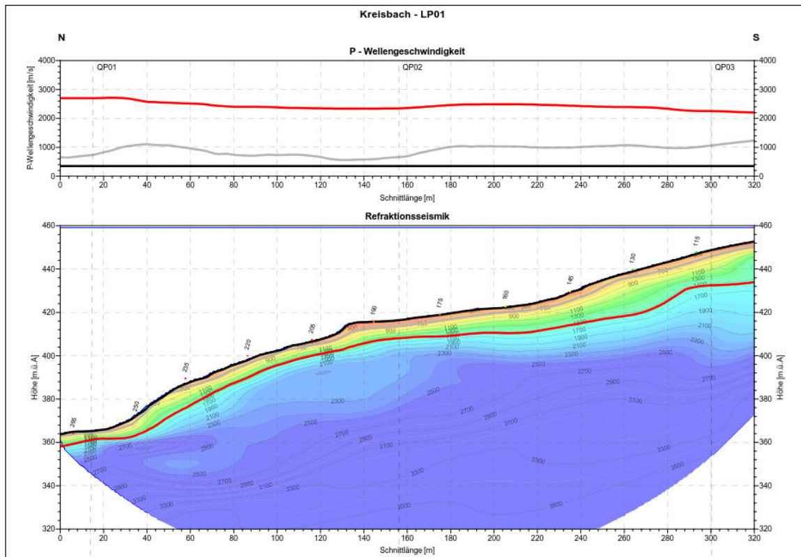
Abb. 7: Seismischer 2D Schnitt entlang des Profils K-LP01
