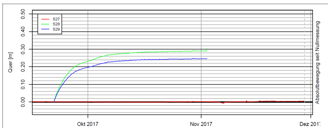
Abb. 10: Querverformungen der Punkte S27 bis S29 beim Monitoring
