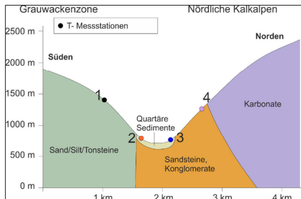
Abbildung 1: Setup der Temperatur Messstationen in Leogang, Salzburg.
