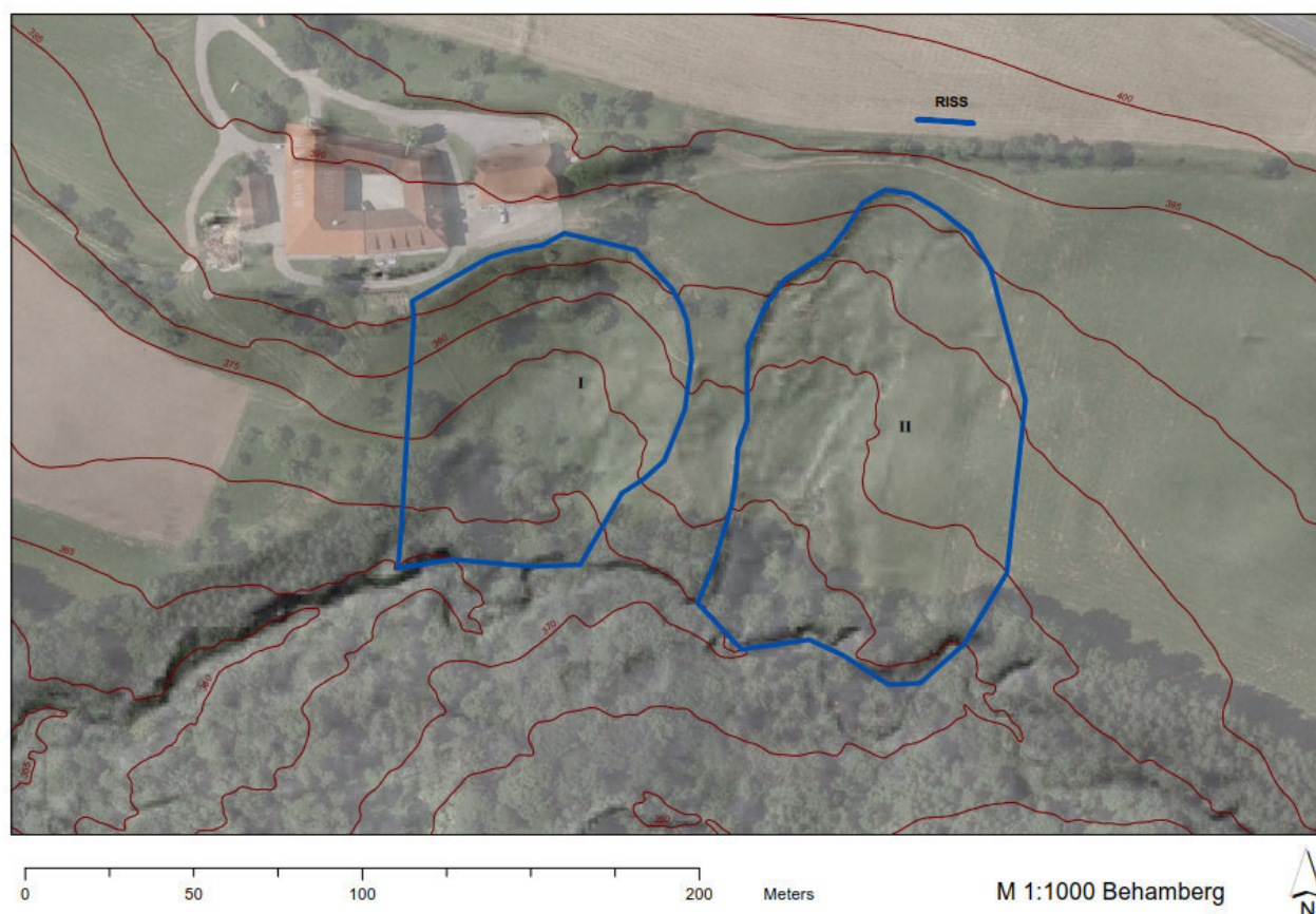
Abb. 5: Rutschung Schweinschwaller, Behamberg, mit zwei Rutschflächen und Bodenriss
