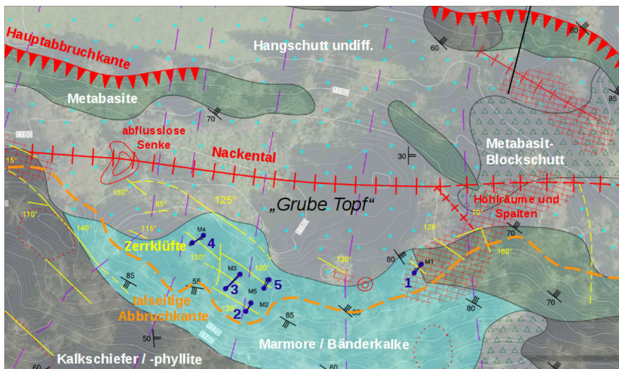
Abb. 5: Geologische Karte des oberen Abschnitts im Ablösebereich West mit Zerrstrukturen und Messstrecken (blau).
