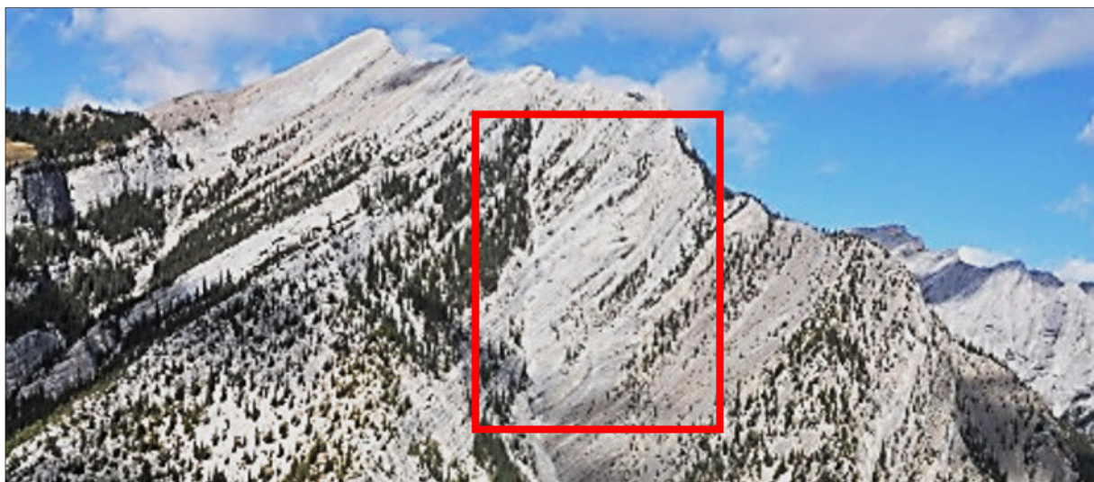
Abb.5: Ansicht der potenziellen Felsgleitung (Foto von M. Jakob, BGC, 2014)
