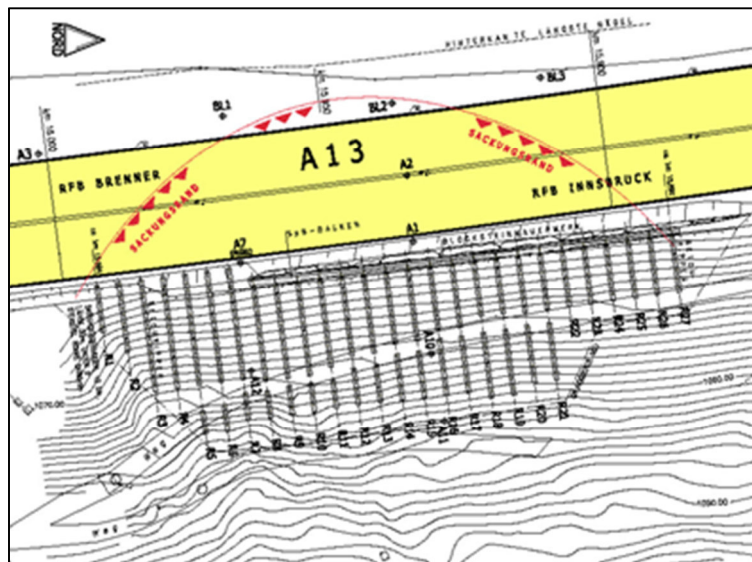
Abb. 4: Anordnung der Hangverdübelung 2005, Grundriss
