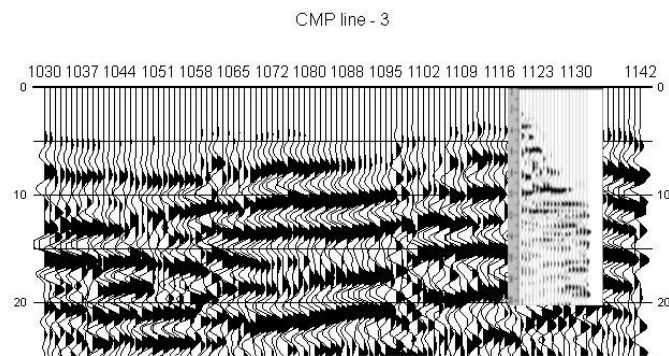
Abb. 9: Offsetbeschränktes tiefengewandeltes Stapelergebnis des Profils BS 3 mit Tiefen-Seismogramm des VSP 2.
