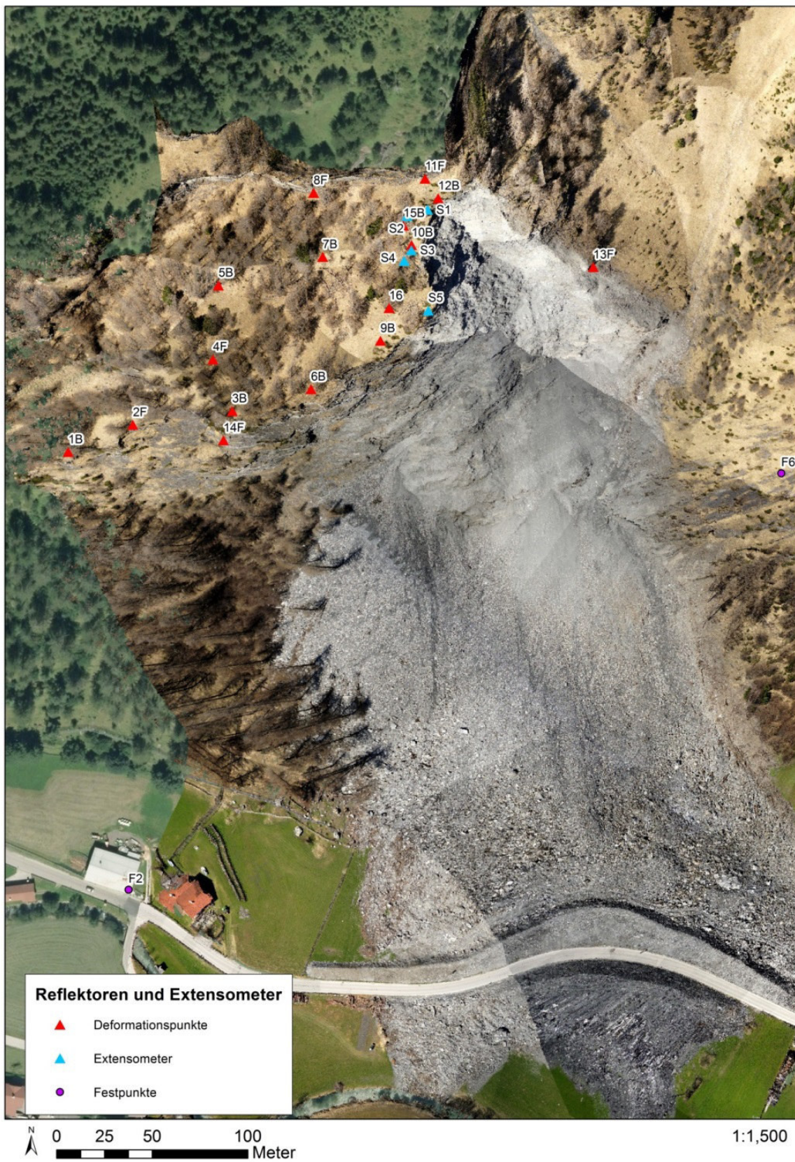
Abbildung 9: Lageübersicht der installierten Reflektoren (rot) und Extensometer (blau)
