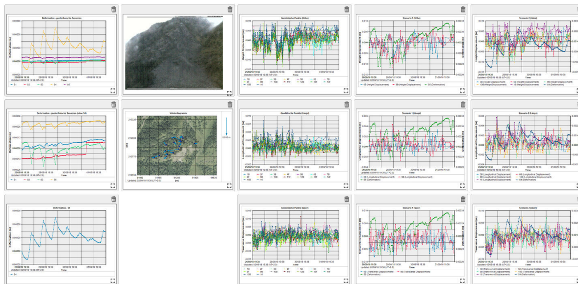
Abbildung 10: Darstellung Leica GeoMos Now
