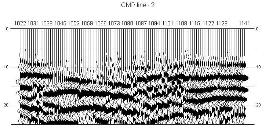
Abb. 8: Offsetbeschränktes, tiefengewandeltes Stapelergebnis des Profils BS 2.
