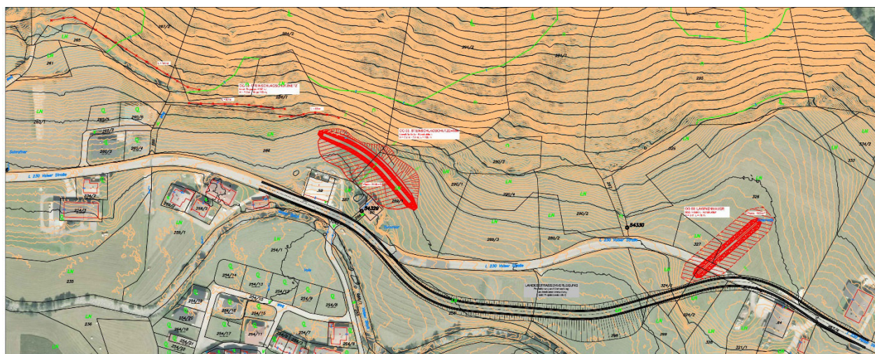
Plan der endgültigen Schutzdammmaßnahmen und der Errichtung neuer Steinschlagschutznetze der WLW für den Siedlungsraum
