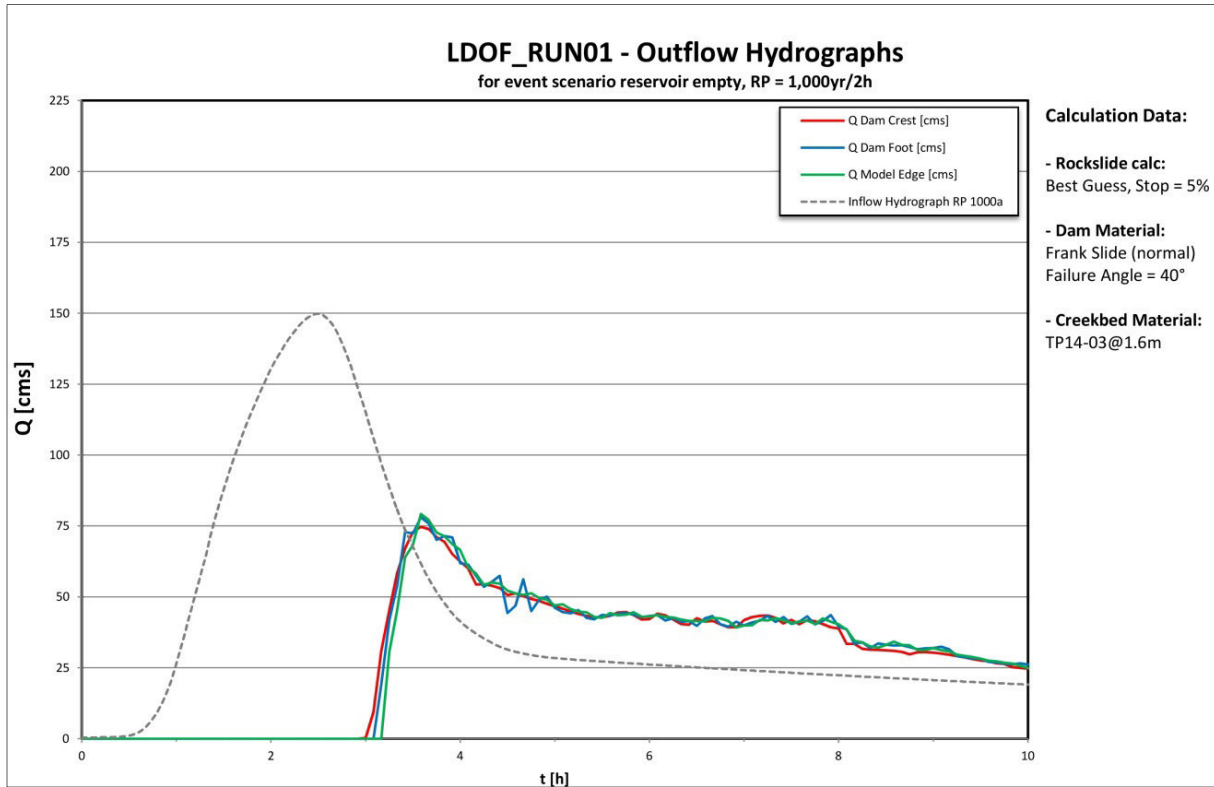
Abb.9: Dambruchhydrograph – Parametersatz 01
