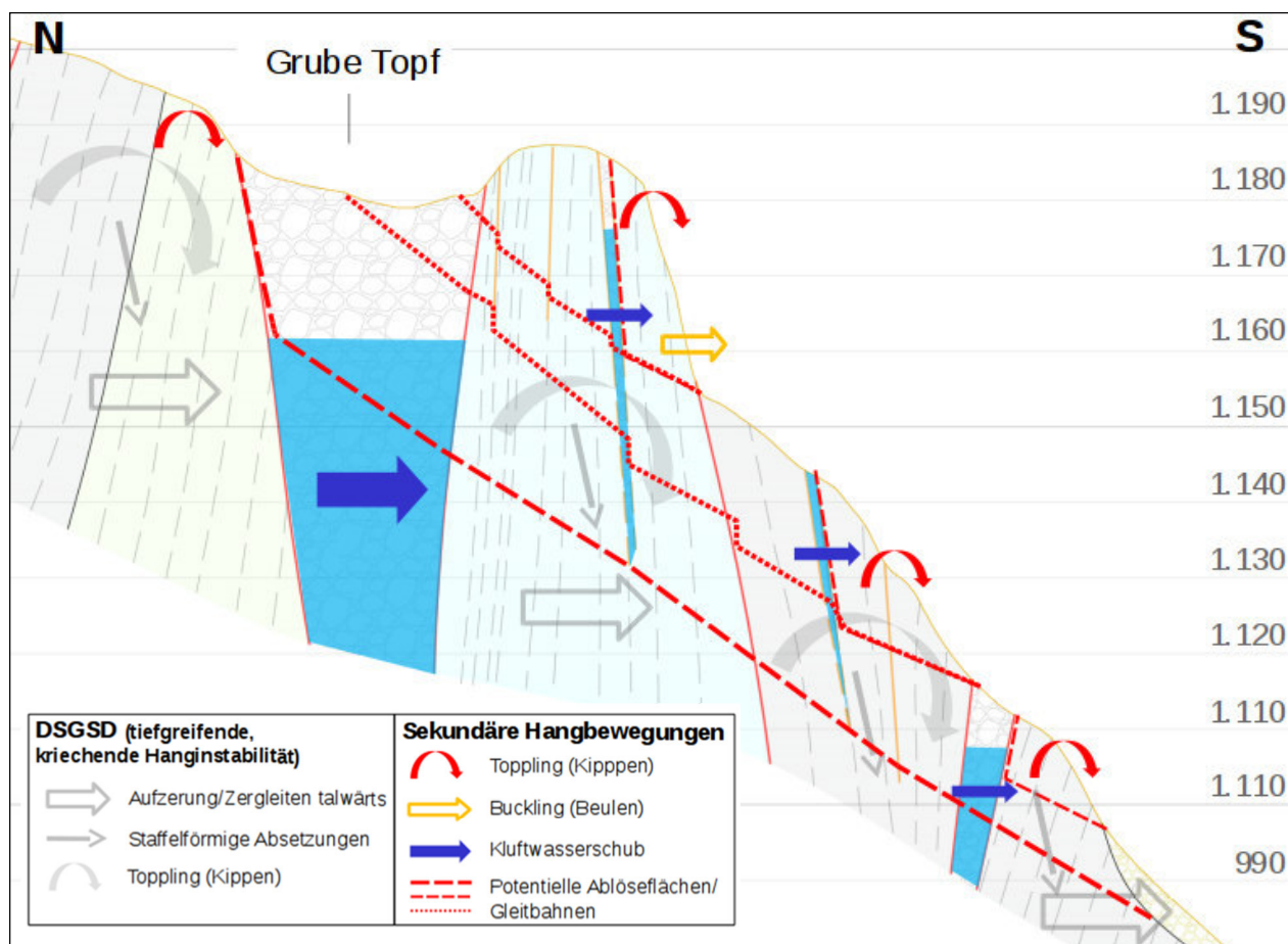
Abb. 9: Schematische Skizze zu den ablaufenden Hangbewegungsprozessen im Ablösebereich West mit Differenzierung zwischen den übergeordneten langsamen Bewegungen (DSGSD) und Ablösemechanismen der sekundären Hangbewegungen.
