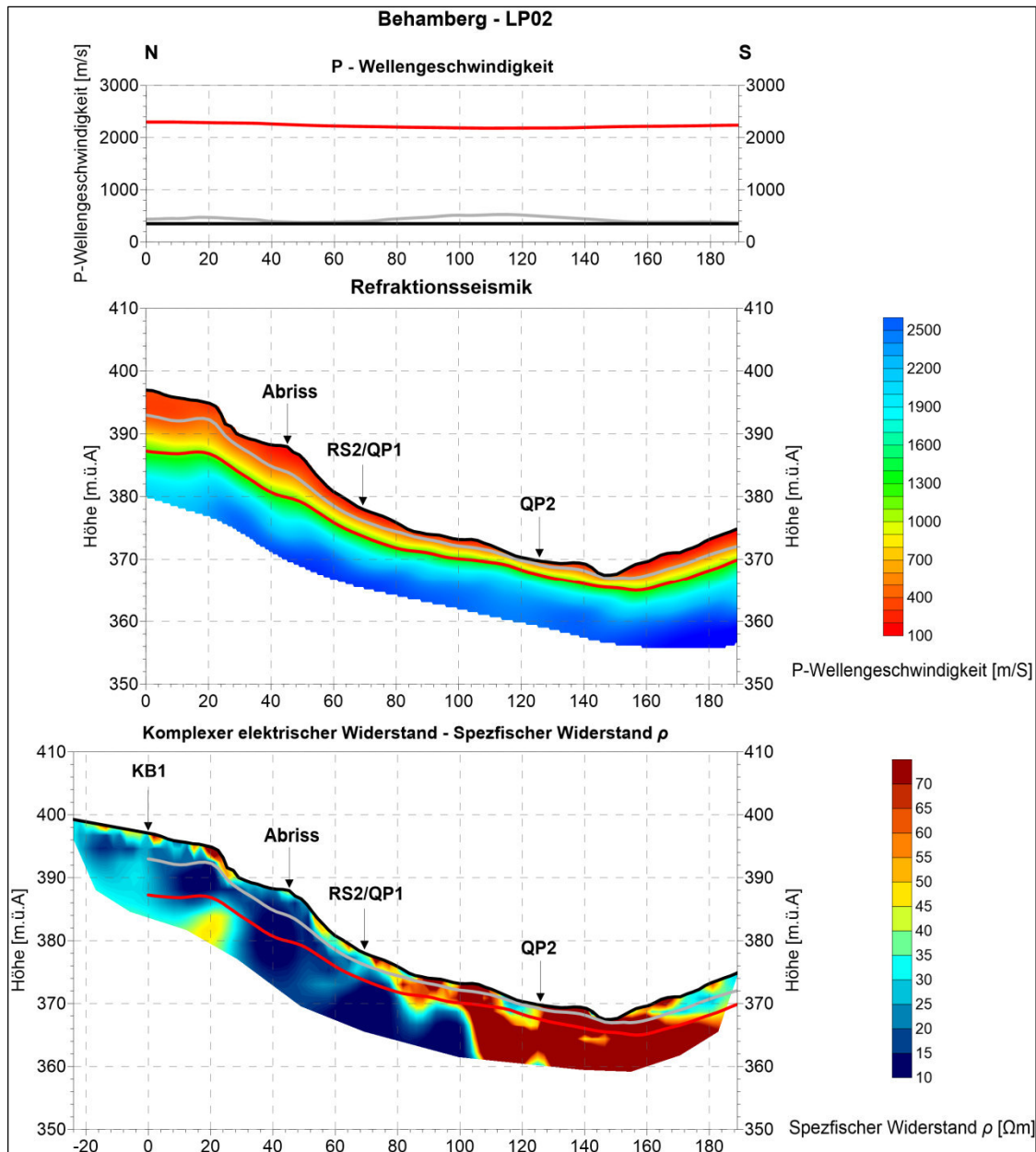
Abb. 10: Geophysikalischer 2D Schnitt entlang von Profil LP02; oben Seismik unten Geoelektrik
