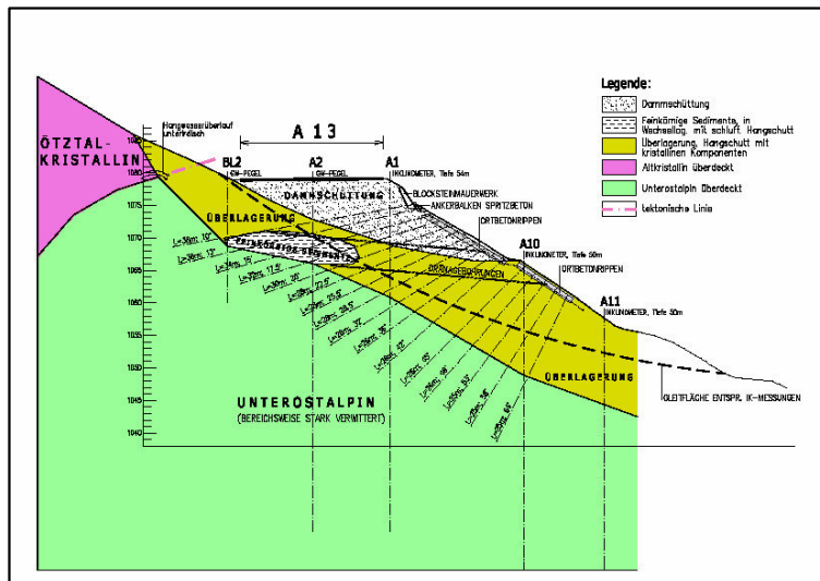
Abb. 3: Geologisches Profil 3 durch Autobahn mit Maßnahmen, Nägeln und Stahlbetonrippen
