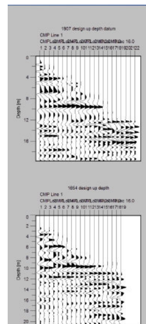
Abb. 4: Seismogramme der aufwärts laufenden Wellenfelder von VSP 1 (oben) bzw. VSP 2 (unten) nach Tiefenwandlung.
