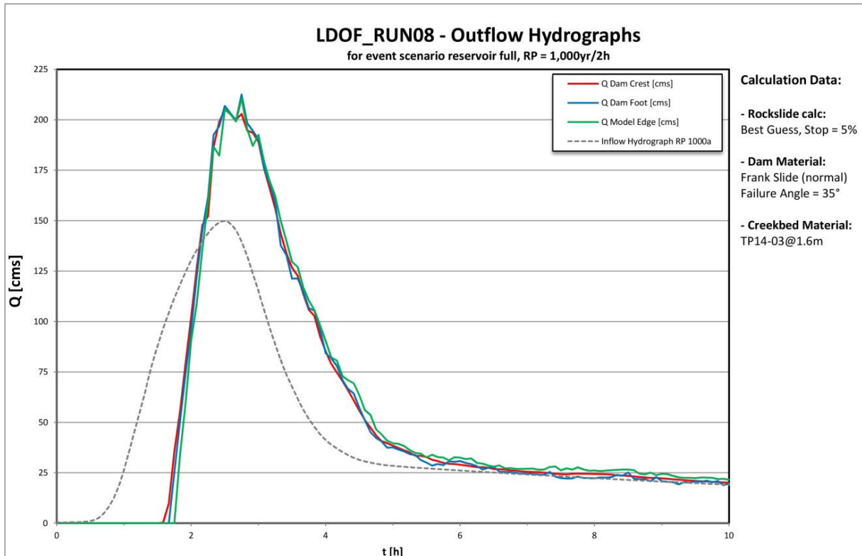
Abb. 10: Dambruchhydrograph – Parametersatz 08
