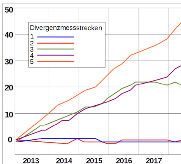
Abb. 6: Divergenzmessungen im Zeitraum 12-2012 bis 06-2018, Verformung in mm.
