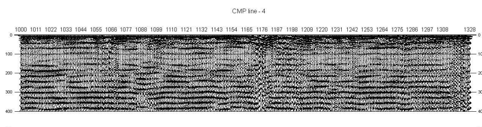
Abb. 2: Stapelergbnis des Profils BS 4 nach konventioneller Bearbeitung.
