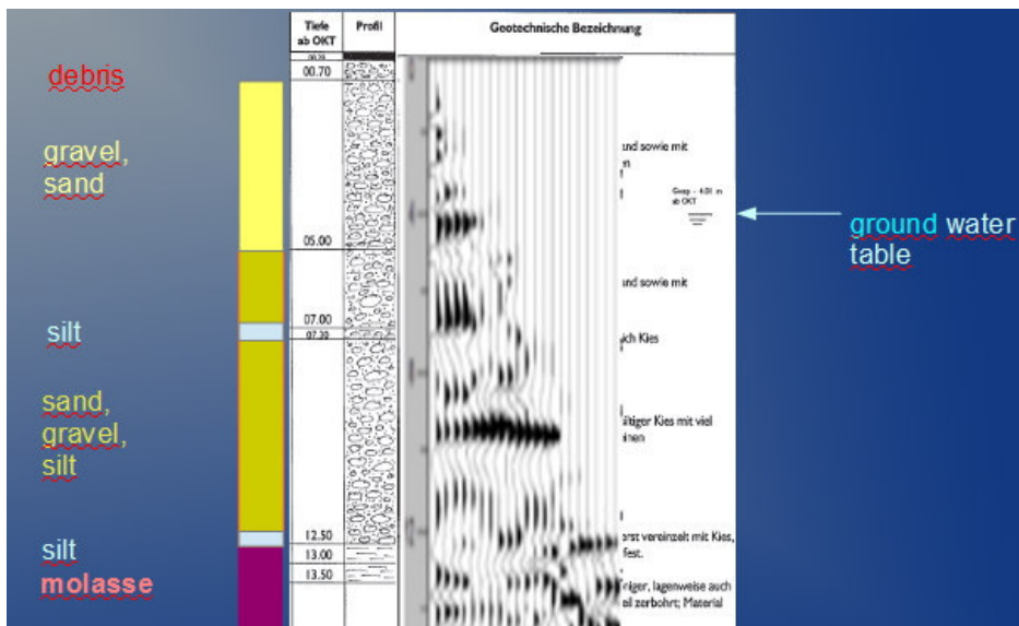
Abb. 10: Teufenabgleich des geologischen Aufschlusses 1907 mit dem VSP1-Ergebnis.
