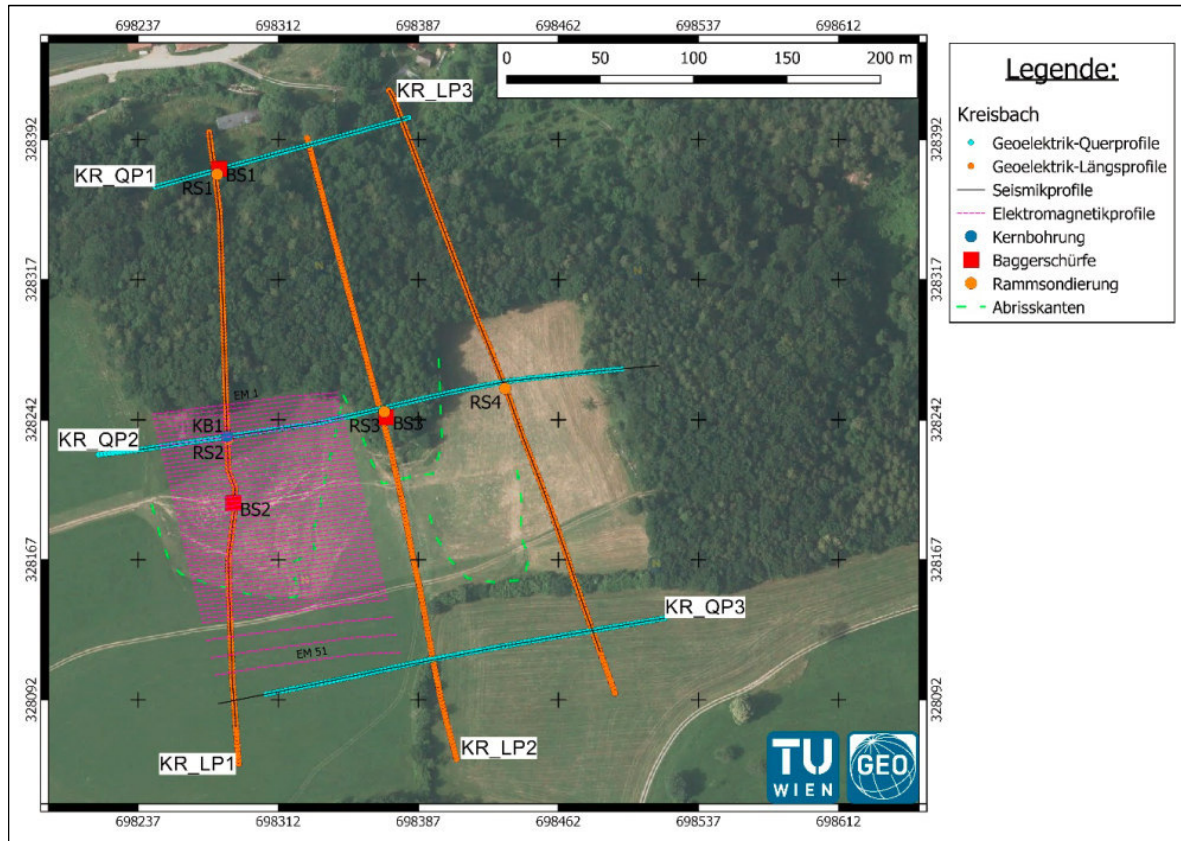
Abb. 6: Lage der geophysikalischen Profile sowie der weiteren Erkundungsmaßnahmen bei der Rutschung „Daxböck“
