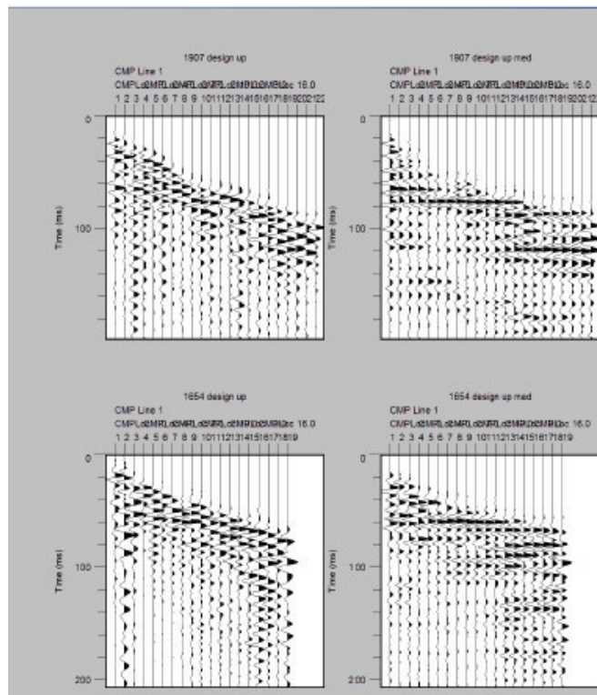
Abb. 3: Seismogramme, Spalte 1: Separierte abwärts laufende Wellenfelder von VSP 1 bzw. VSP 2. Spalte 2: Separierte aufwärts laufende Wellenfelder der VSP .
