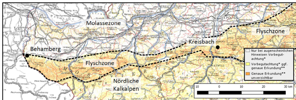
Abb. 1: Die zwei Untersuchungsgebiete in der Flyschzone (der in Niederösterreich gelegene Teil der Flyschzone ist durch die gestrichelte Linie hervorgehoben) und in der nördlich davon gelegenen Molassezone. Die Hintergrundkarte (Quelle: Land Niederösterreich, NÖ Atlas 4.0) gibt Handlungsempfehlungen bei Rutschprozessen an (siehe Legende).
