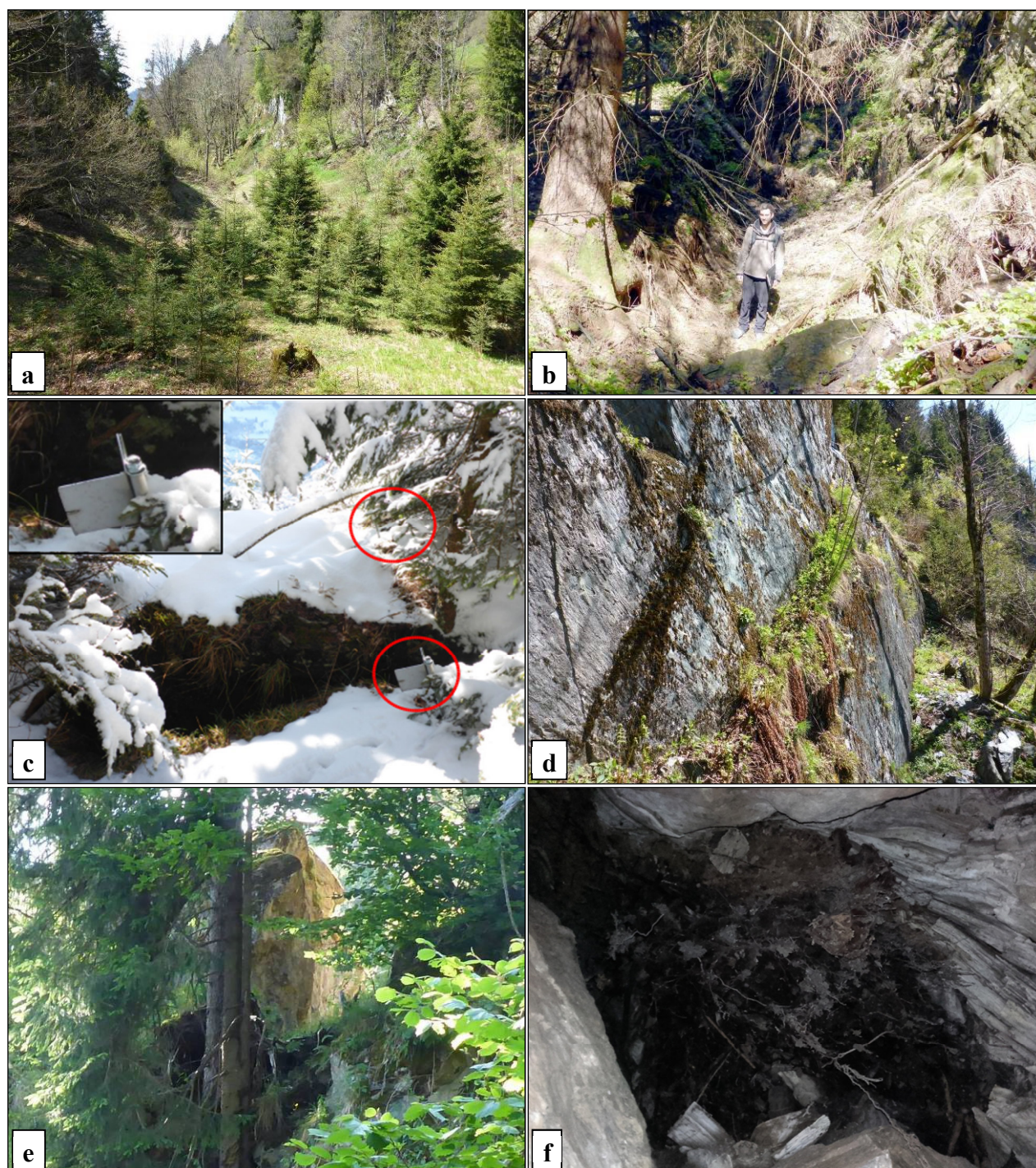
Abb. 8: Unterschiedlich große Zerrstrukturen im Ablösebereich West mit dem Nackental "Grube Topf" (a), einem kleinen Nackental am Hang darüber (b) und einer geöffneten Kluft mit rot markierten Anschlagpunkten der Divergenzmessstrecke 2 und Detail eines Anschlagpunktes (c). Bergseitige Begrenzung des Nackentales im Ablösebereich Ost mit steil stehender Störungsfläche in Metatuffiten (d). Isolierter Felsblock im bewaldeten Unterhang des Ablösebereiches West (e). Blick nach oben auf den Waldboden in einer verwachsenen begehbaren Spalte (f).
