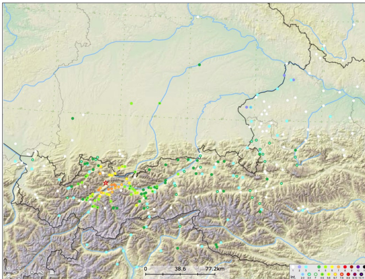
Abb. 5: Nassereith Beben vom 13. Juli 1910. Die Karte zeigt die Verteilung der 269 IDPs. Der Stern markiert das Epizentrum des Bebens in Nassereith.
