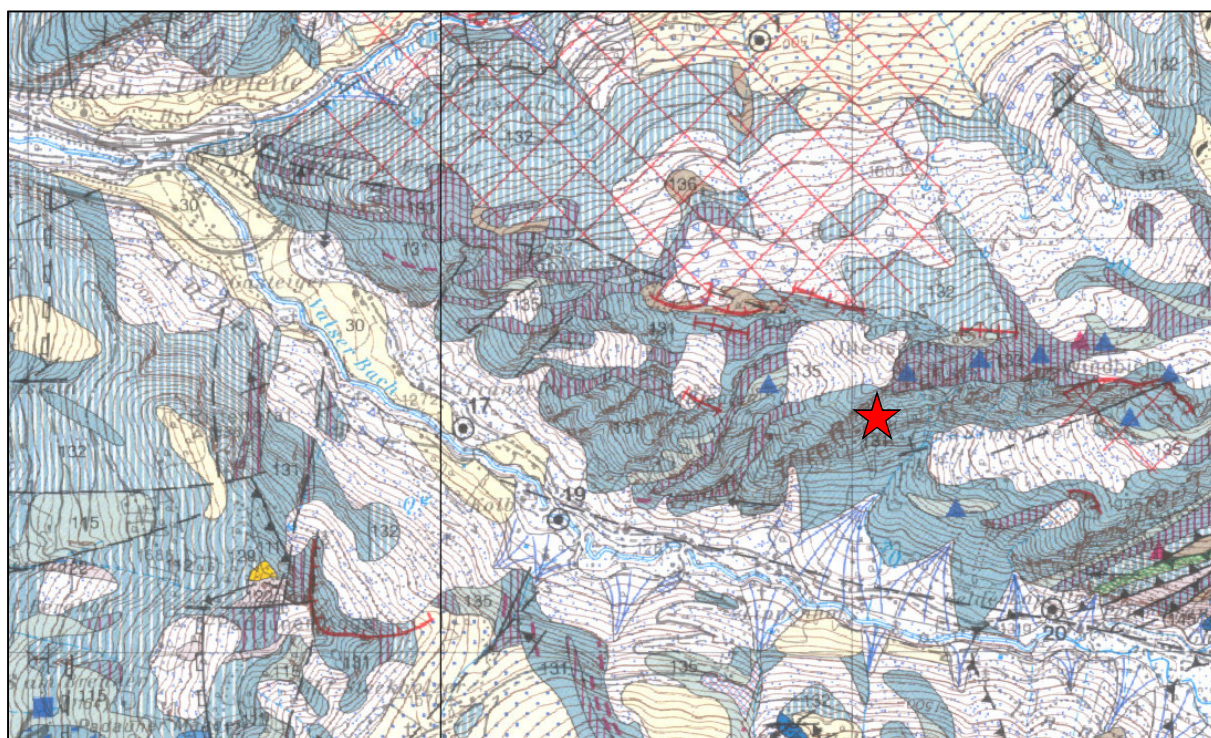
Abb.1. Ausschnitt Geofast/GBA – geologische Karte. Der rote Stern markiert die Stelle der Sturzwand
