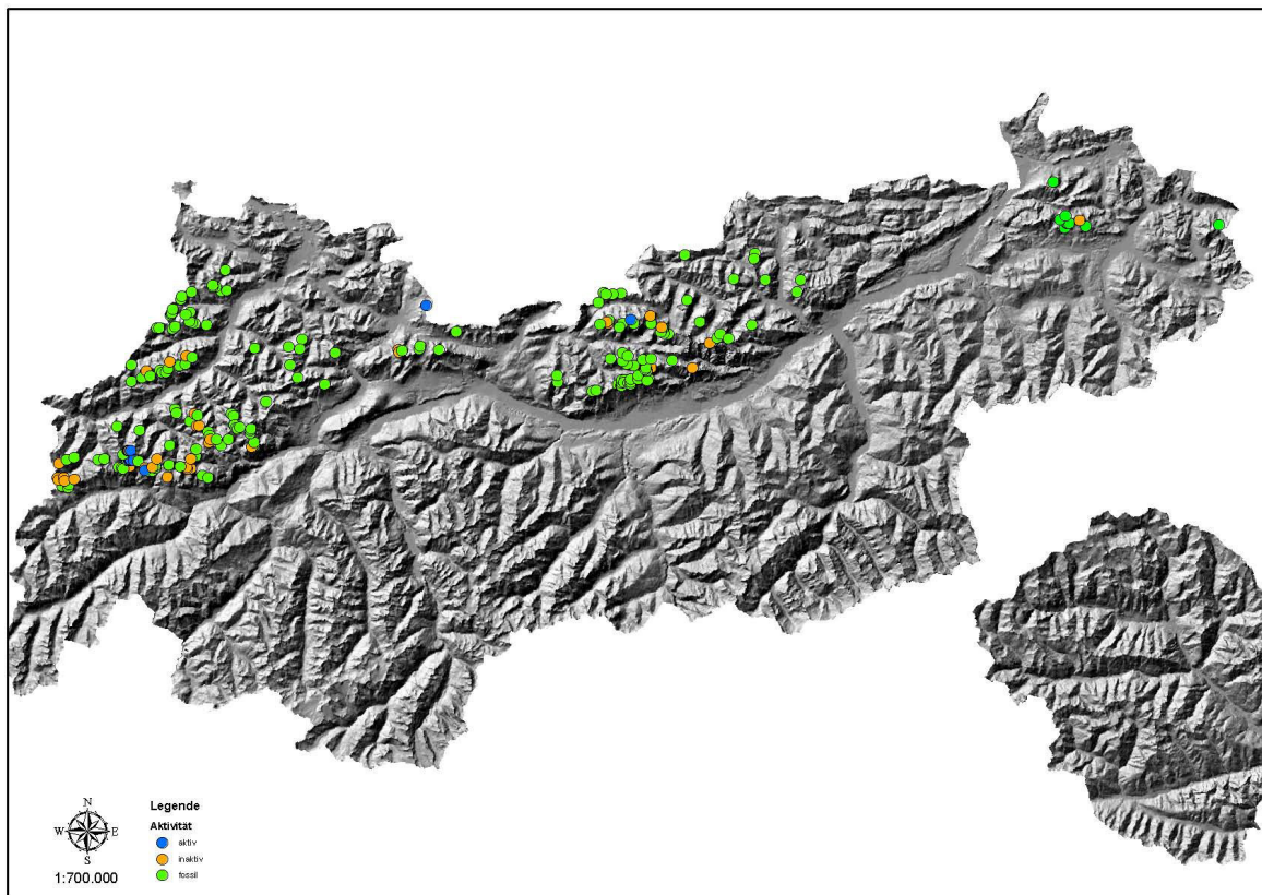
Abb. 1: Verbreitung der Blockgletscher in den Nördlichen Kalkalpen
