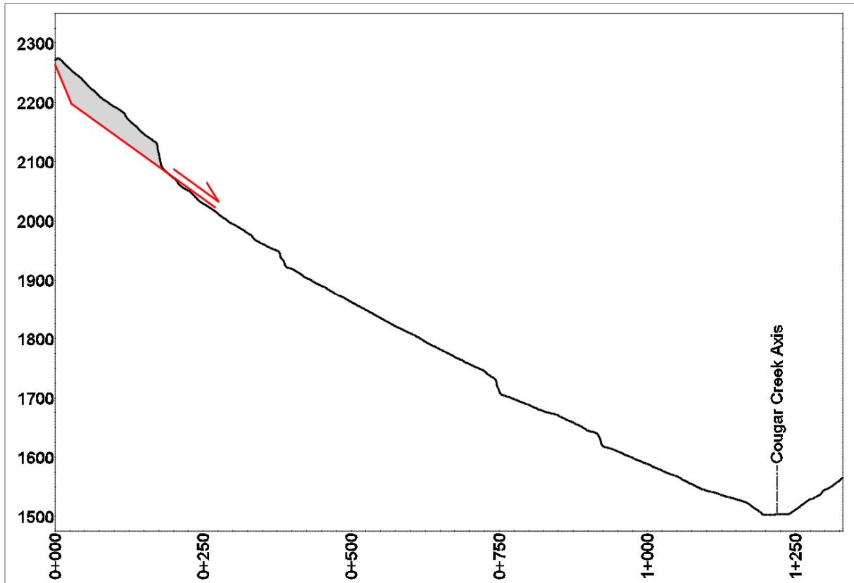
Abb.4: Längenschnitt durch die potenzielle Sturzbahn samt Ablöseform
