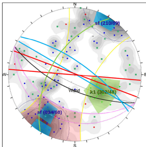
Abb. 3: Polpunkte der 137 Feldmessungen mit den wichtigsten strukturgeologischen Elementen als Großkreise (Schieferung, Klüftschar k1, Störungen, Steilwand Ablösebereich West). Der rötliche Bereich repräsentiert die kritische Polpunktzone aus einer kinematischen Analyse für Flexural Toppling (Hangneigung > 50°).
